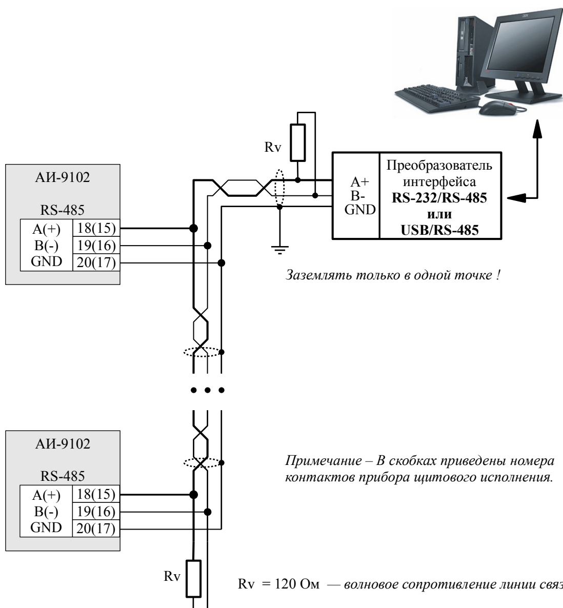
Рисунок В.5 Включение анализаторов в локальную сеть Modbus.
