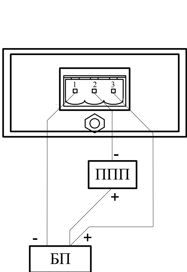
Рисунок В.1 - Подключение пассивного первичного преобразователя (ППП)
